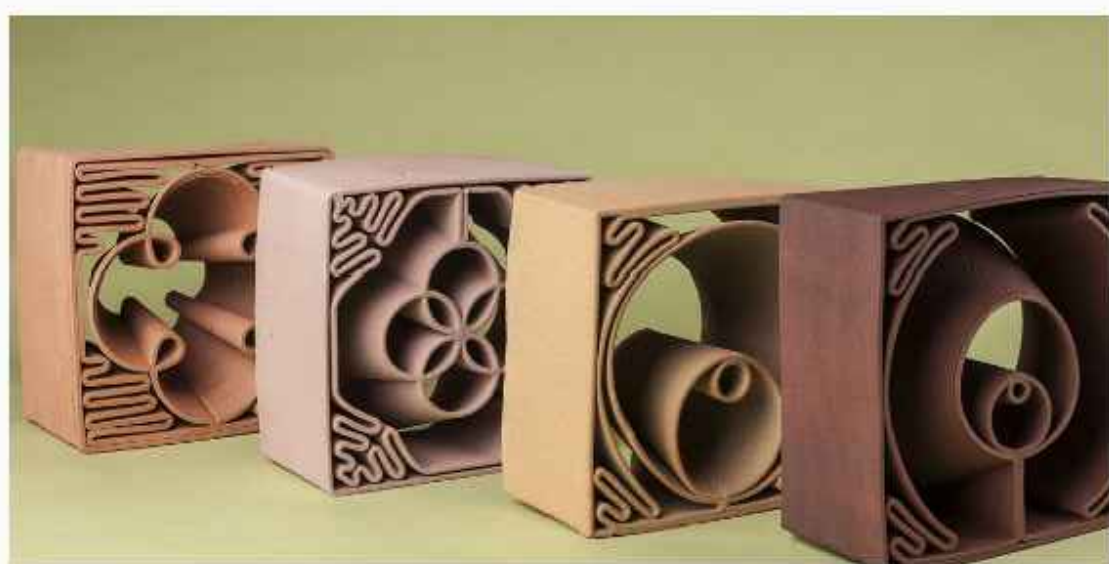
© Ultra Ordinaire, Low-tech ventilation system, Prototype design - Nathalie Bruyère & Pierre Duffau. Production prototype - 8FabLab. Source : https://ultra-ordinaire.com/en/
